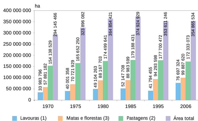
Gráfico 1 - Utilização das terras - Brasil - 1970/2006
