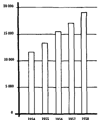
PRODUÇÃO (1 000 000 kW)
