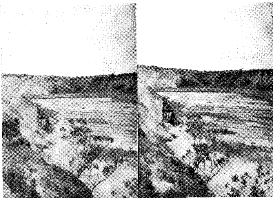
Fig. 3 — Par estereoscópico a jusante do ribeirão Saboeiro, mostrando em 1, o cotovêlo de captura; e o aspecto das voçorocas nas imediações da mesma
