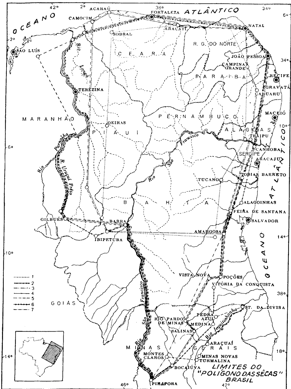
Fig. 1 — Aumento progressivo da área oficialmente reconhecida como das sêcas. Nota-se a superposição com o Vale do São Francisco, e para o desenvolvimento desta região o governo federal aplicará uma verba tributária nunca inferior a 1%. (Geography's Contribution to the Better Use of Resources — HILGARD O'REILLY STENBERG).
