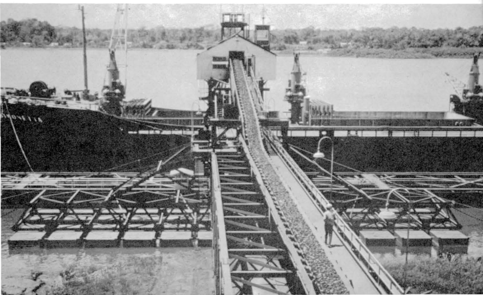
Macapá — Porto de Santana Esteira para o transporte de manganês
