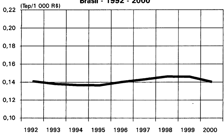
Gráfico 47 - Intensidade energética Brasil - 1992 - 2000
