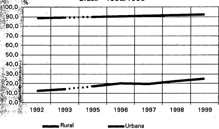
Gráfico 36 - Percentual de moradores em domicílios particulares permanentes com acesso a sistema de abastecimento de água, segundo situação do domicílio Brasil - 1992/1999
