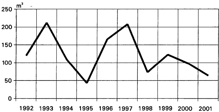
Gráfico 53 - Produção de rejeitos radioativos de baixo e médio nível de atividade da Usina Nuclear de Angra I Brasil - 1992 - 2001
