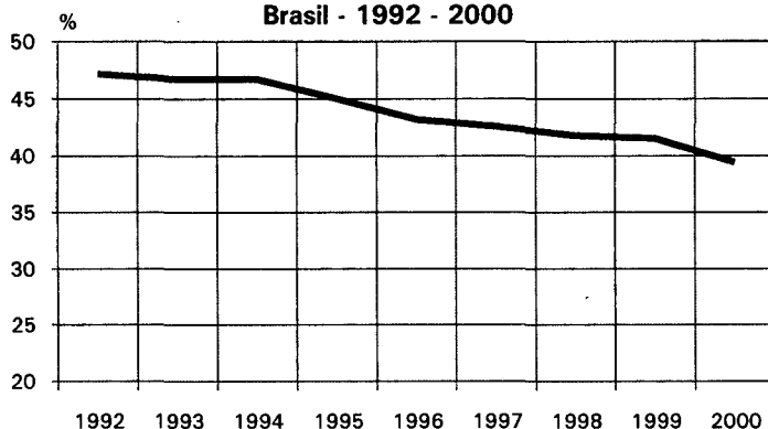
Gráfico 48 - Participação de energia renovável sobre o total de energia ofertada Brasil - 1992 - 2000
