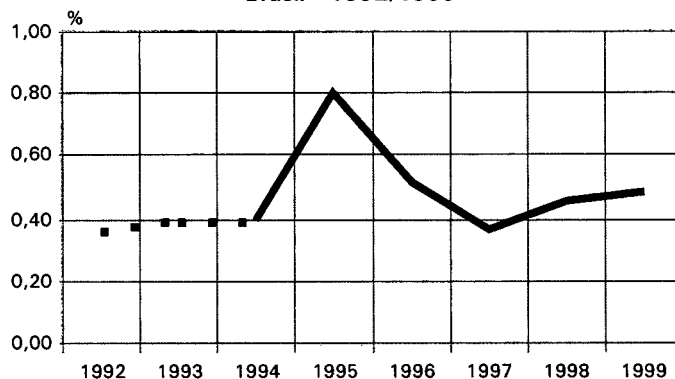
Gráfico 27 - Taxa de desflorestamento bruto anual em relação à área de floresta remanescente na Amazônia Legal Brasil - 1992/1999
