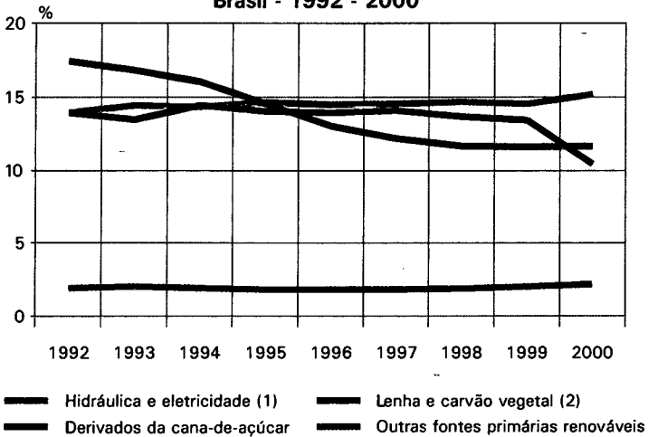
Gráfico 50 - Participação das fontes renováveis no total de energia ofertada Brasil - 1992 - 2000
