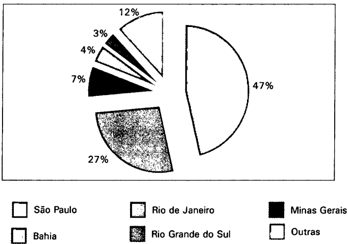
Gráfico 52 - Distribuição percentual dos rejeitos nos depósitos da CNEN, por Unidades da Federação de origem Brasil - 2001
