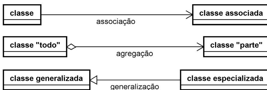
Figura 2 - Notação dos relacionamentos: associação, agregação e generalização
