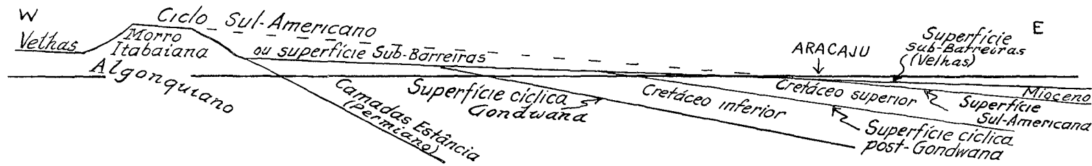
Fig. 8 — Seção esquemática entre Aracaju e Itabaiana, Sergipe mostrando as relações entre as series sedimentares e as superficies ciclicas.
